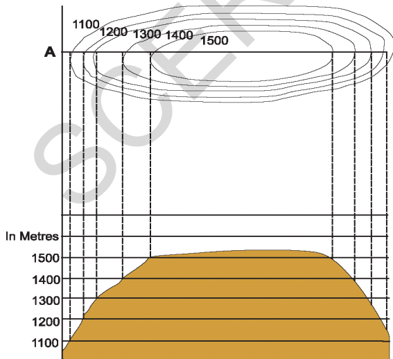
ಚಿತ್ರ 1.10: ಪ್ರಸ್ಥಭೂಮಿ ಕಾಂಟೂರು ರೇಖೆಗಳು
