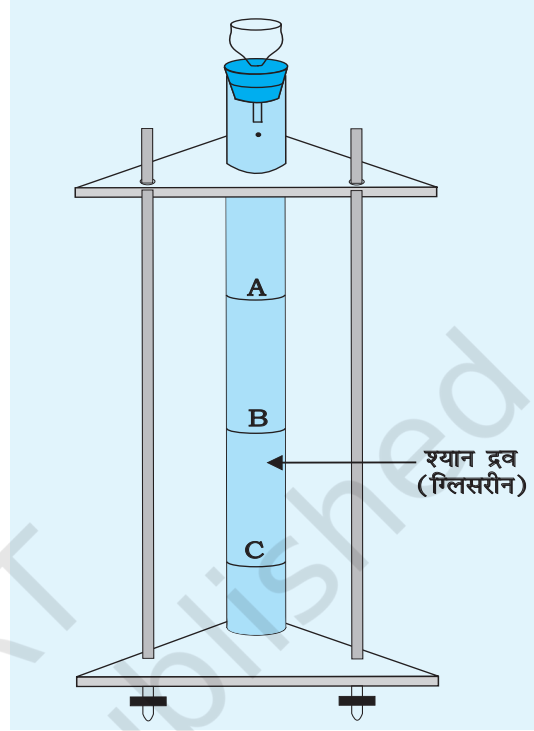
चित्र E 13.3 लंबे ऊर्ध्वाधर नली के अक्ष के अनुदिश सीमांत वेग से गिरती स्टील की गोली
