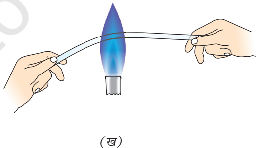
चित्र 2.3 - (क) नली को गरम करना (ख) नली का मुलायम होकर अपने ही भार से मुड़ना (ग) मोड़ को समतलीय करना
