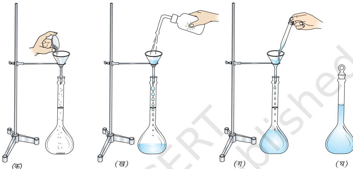
चित्र 2.27 - (क) ऑक्सैलिक अम्ल अंतर्गिरित करना (ख) विलयन का तनुकरण (ग) अन्तिम कुछ mL बूंद-बूंद करके मिलाना (घ) मानक विलयन
